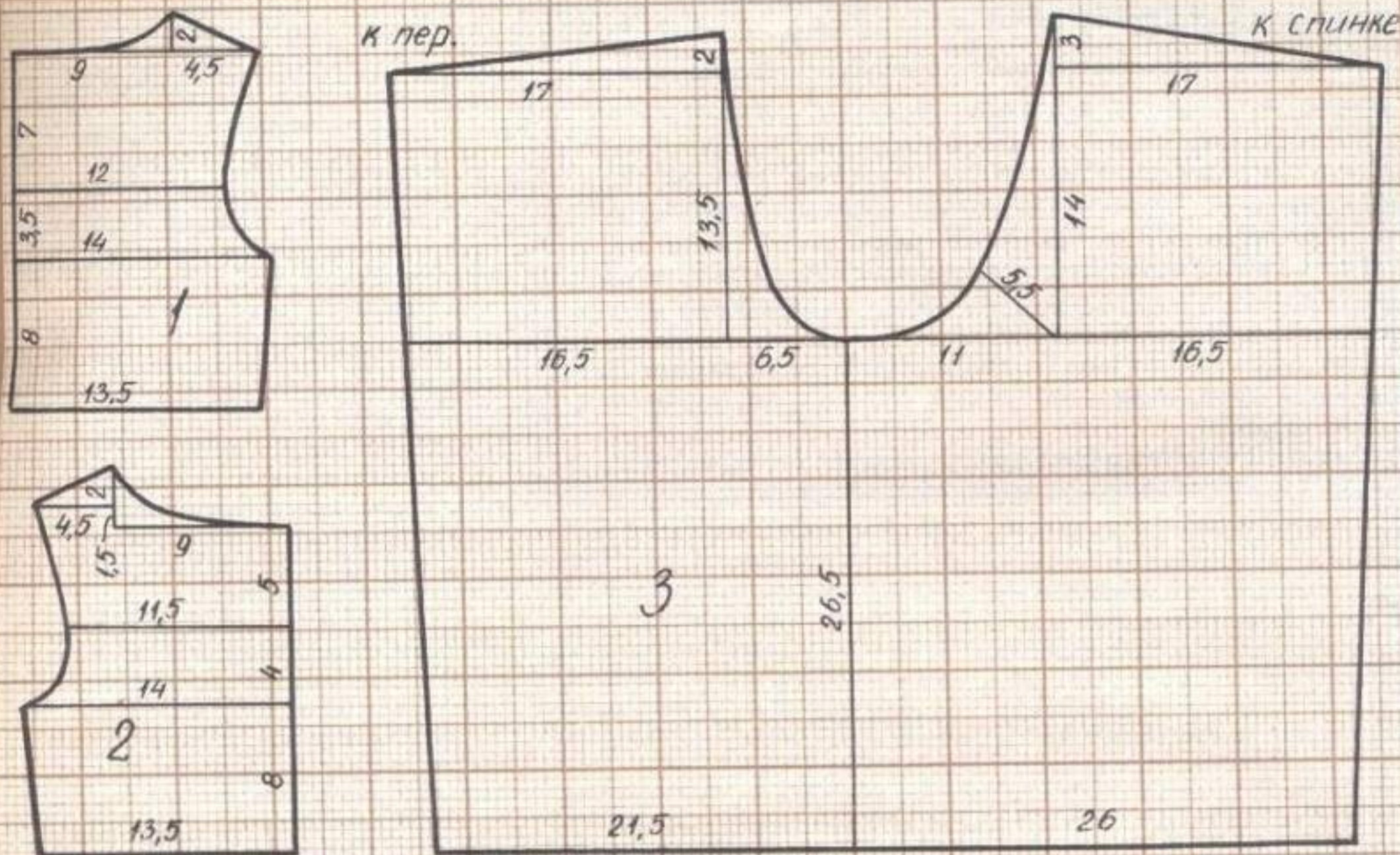
5. Комбинезон из трикотажных полотен. По шву талии притачена узкая резинка. Застежка на глече на навесные петли и пуговицы.
